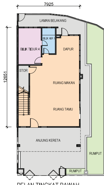
PELAN TINGKAT BAWAH
