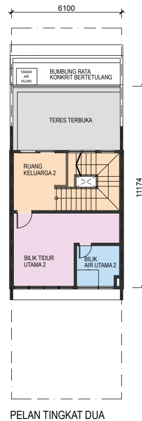
Rumah Teres 3 Tingkat JENIS B 20' x 67.5'
