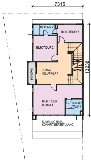
PELAN TINGKAT SATU
