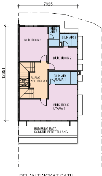
PELAN TINGKAT SATU
