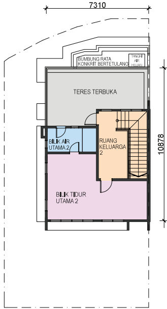
PELAN TINGKAT DUA
