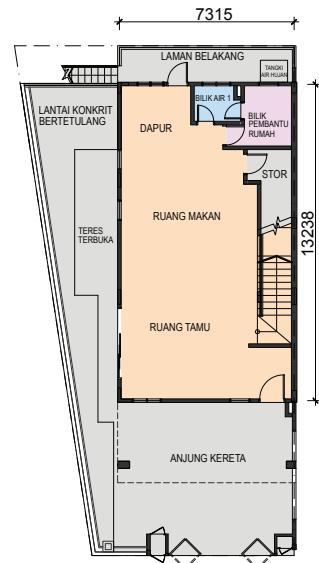
PELAN TINGKAT BAWAH
