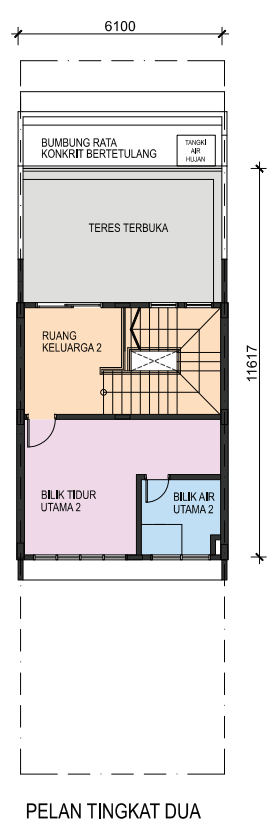
Rumah Teres 3 Tingkat JENIS E 20' x 70'
