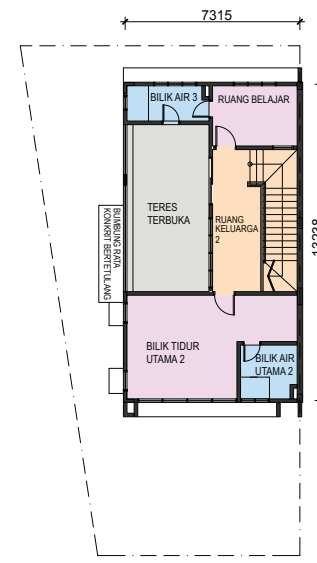
PELAN TINGKAT DUA
