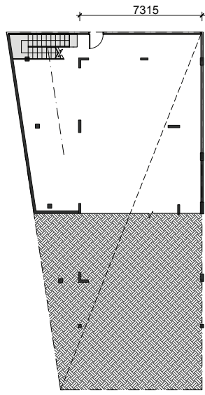
PELAN TINGKAT BAWAH RENDAH
