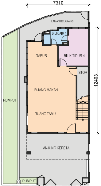
PELAN TINGKAT BAWAH
